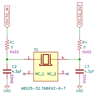
32.768KHZ Crystal
