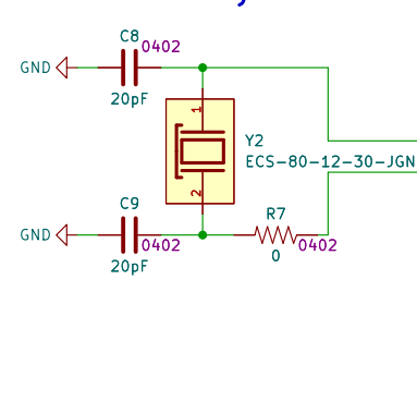
8MHz Crystal
