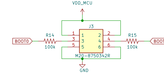
Boot Options
